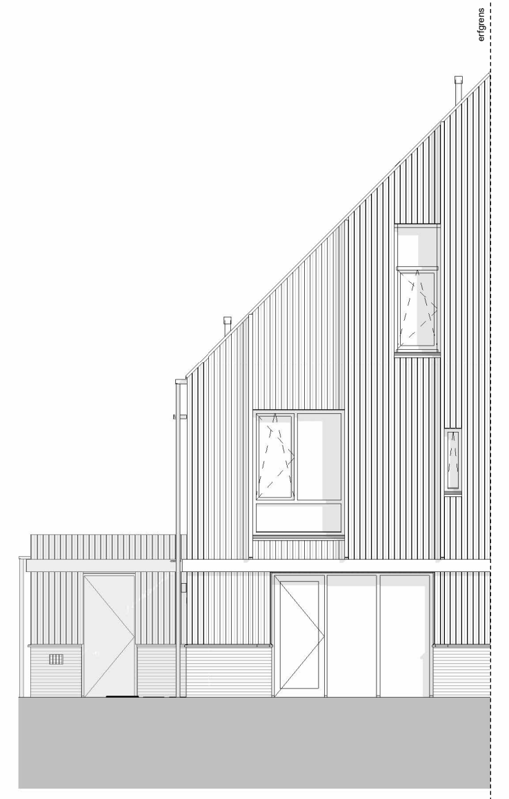
voorgevel (noordoost)
